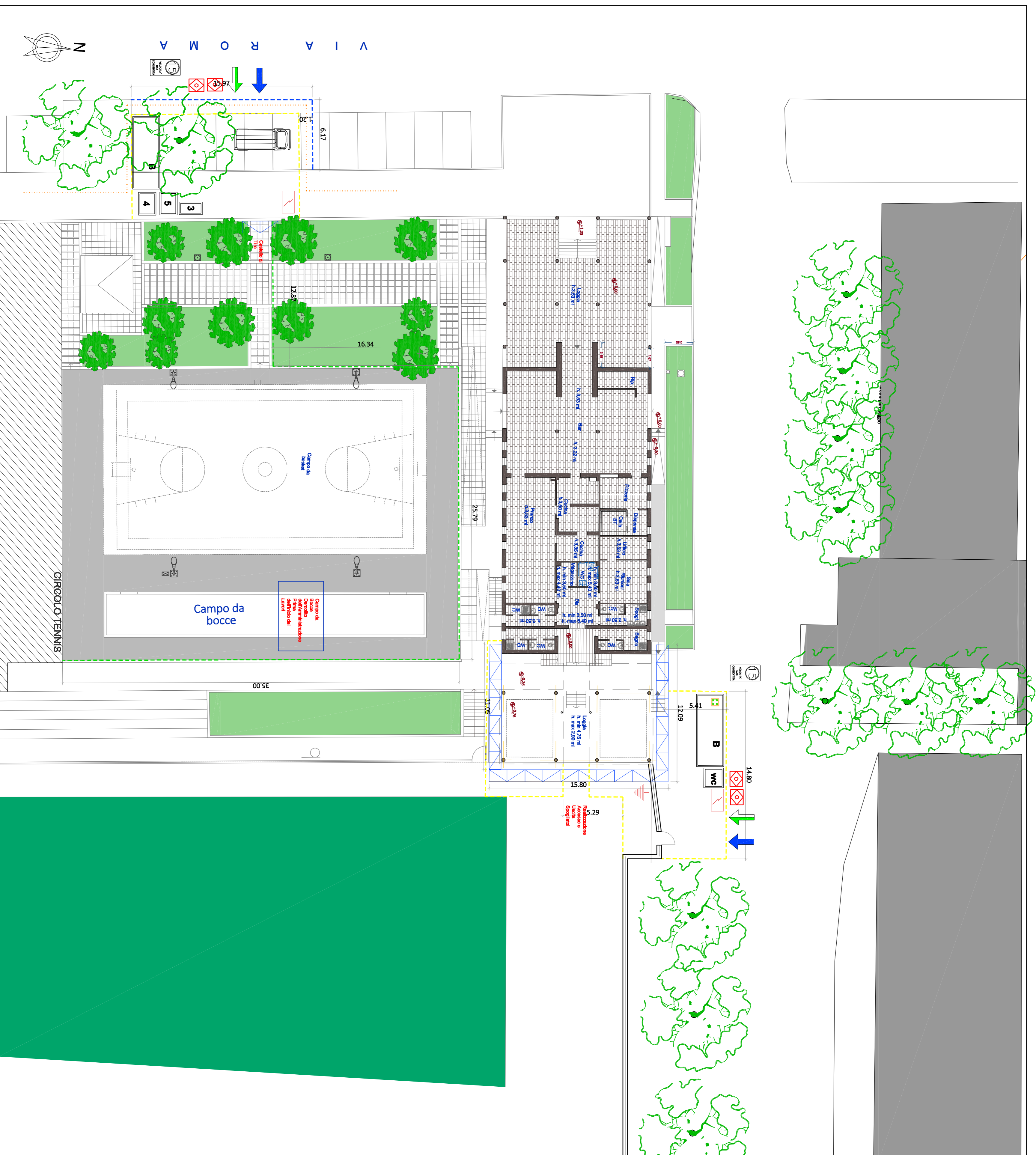
PLANIMETRIA DI CANTIERE
