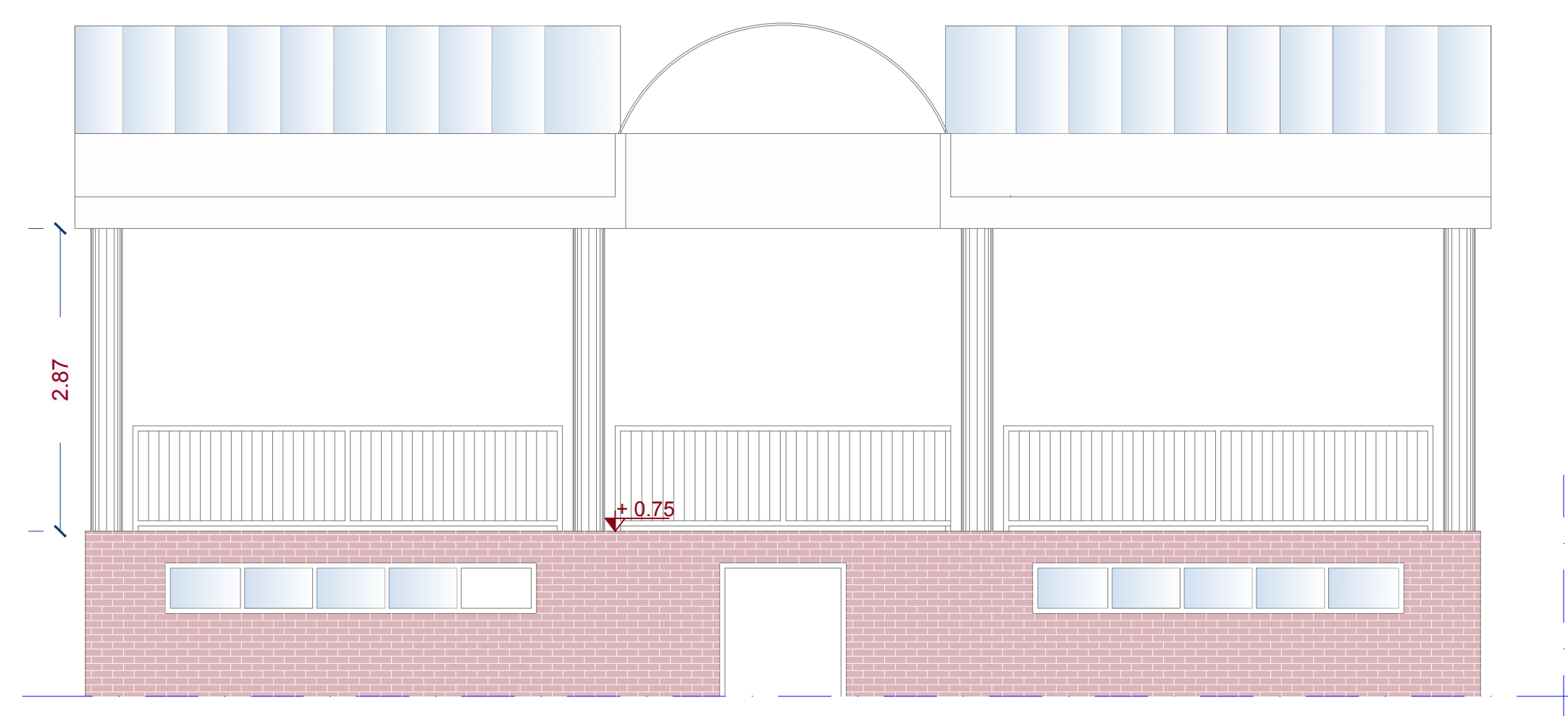
PROSPETTO NORD
