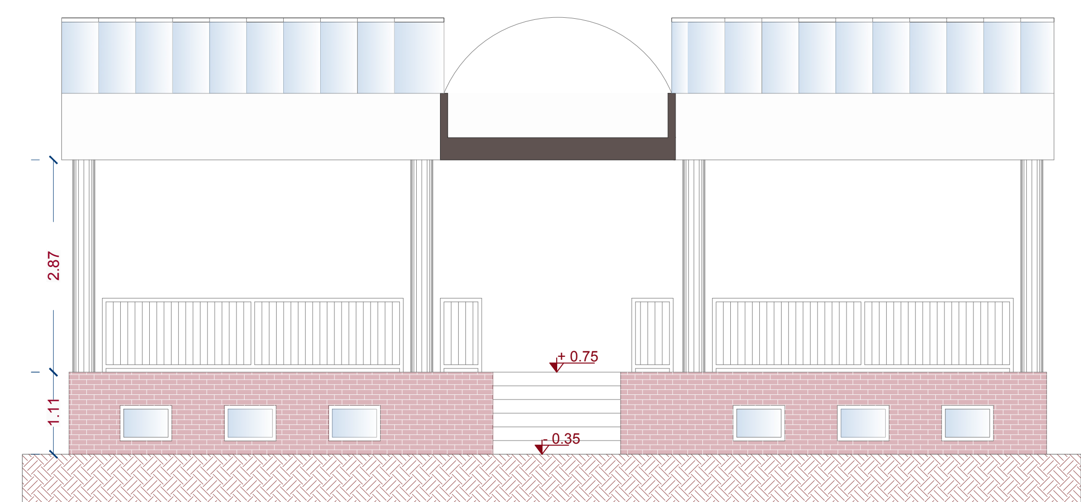
SEZIONE AA'_PROSPETTO OVEST
